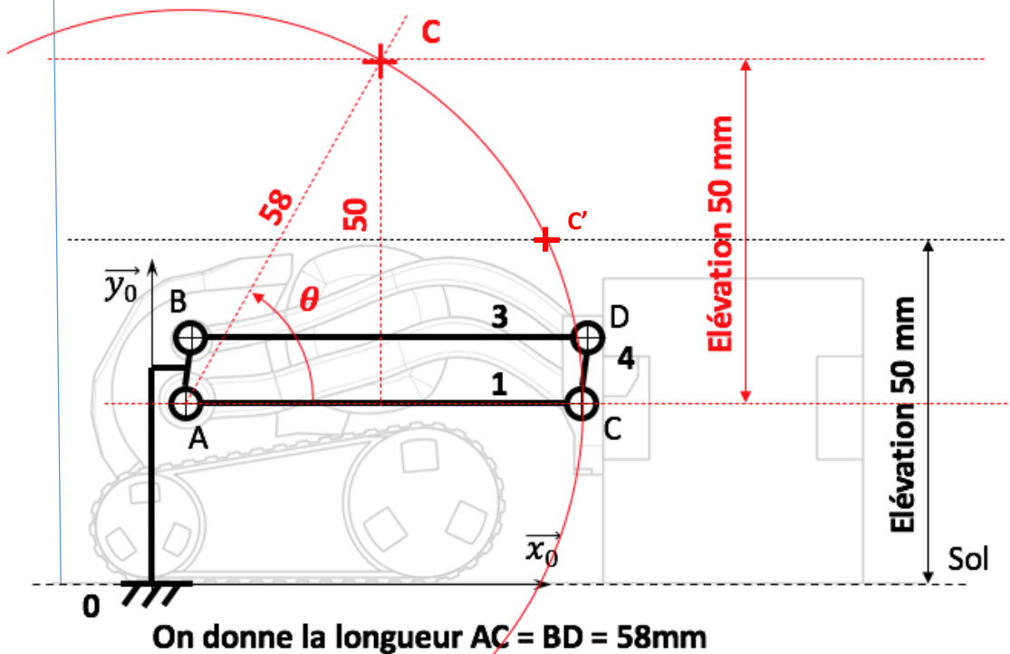
Fig.1 : schéma cinématique
